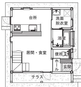
1階平面図
