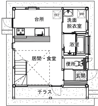
1階平面図
