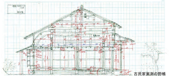
古民家実測の野帳
